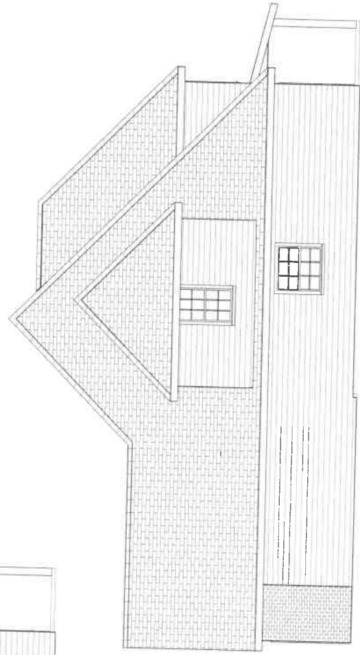
right elevation
